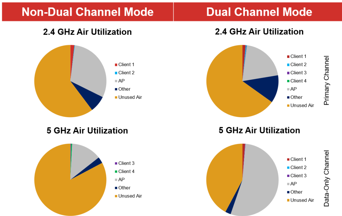
Figure 4 - Scenario A: Airtime Utilization
